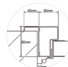
Rėmo matmenys
