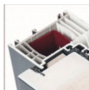
Šešių kamerų PVC stakta
