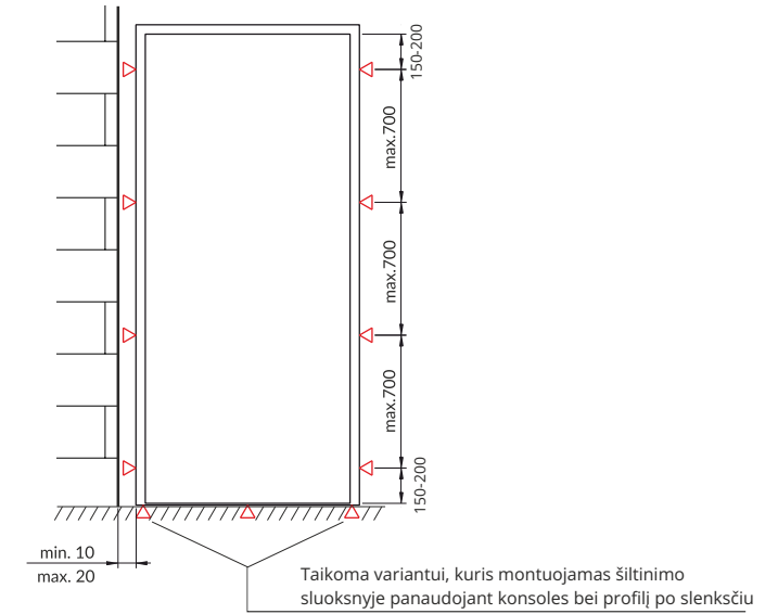
Optimalūs durų bei langelių tvirtinimo punktai
