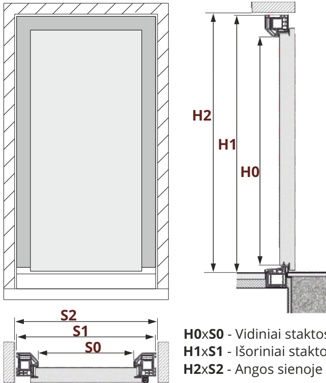
Durų matmenų schema
